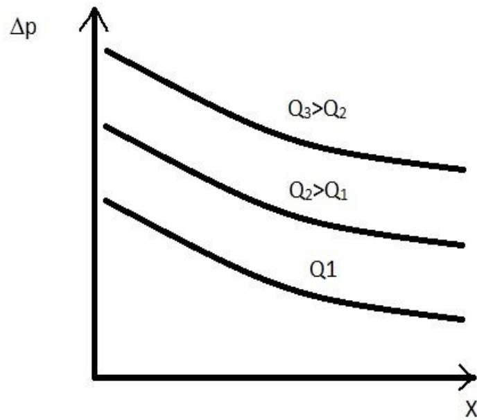
Rys. 2. Wykres zależności \Delta p = f(x) dla rozdzielacza przy różnych wartościach natężenia przepływu
